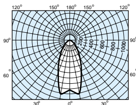
配光曲線圖 RF100V135WHC
