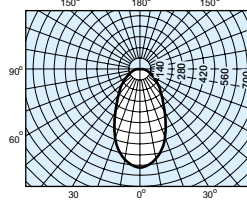
配光曲線圖
