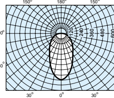
配光曲線圖
