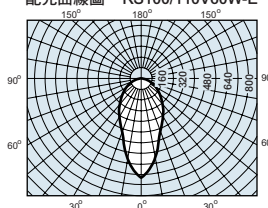
配光曲線圖 RS100/110V60W-E
