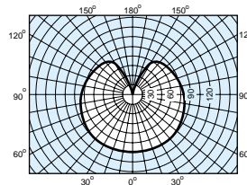
配光曲線圖
