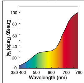
電磁波頻譜圖(Spectral energy distribution graphs)
