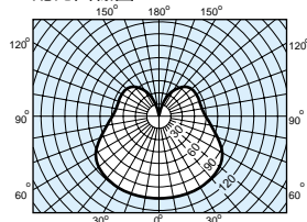
配光曲線圖
