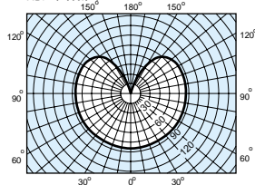
配光曲線圖 LW100V54W55
